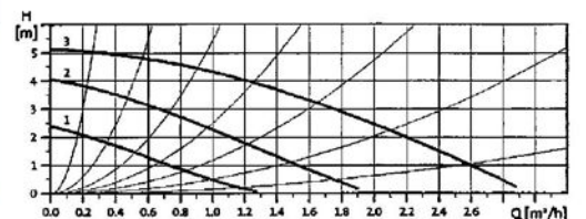
Pompa Basıncı Grafiği
