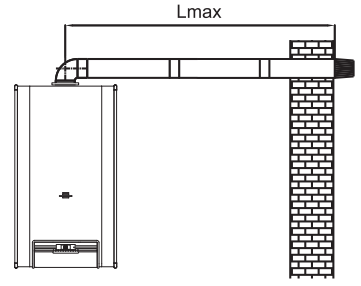
Yatay Hermetik Baca Uygulaması (Tek Dirsekli Lmax. Mesafesi : 3 m, Ø60/100) (Tek Dirsekli Lmax. Mesafesi : 6 m, Ø80/125)
