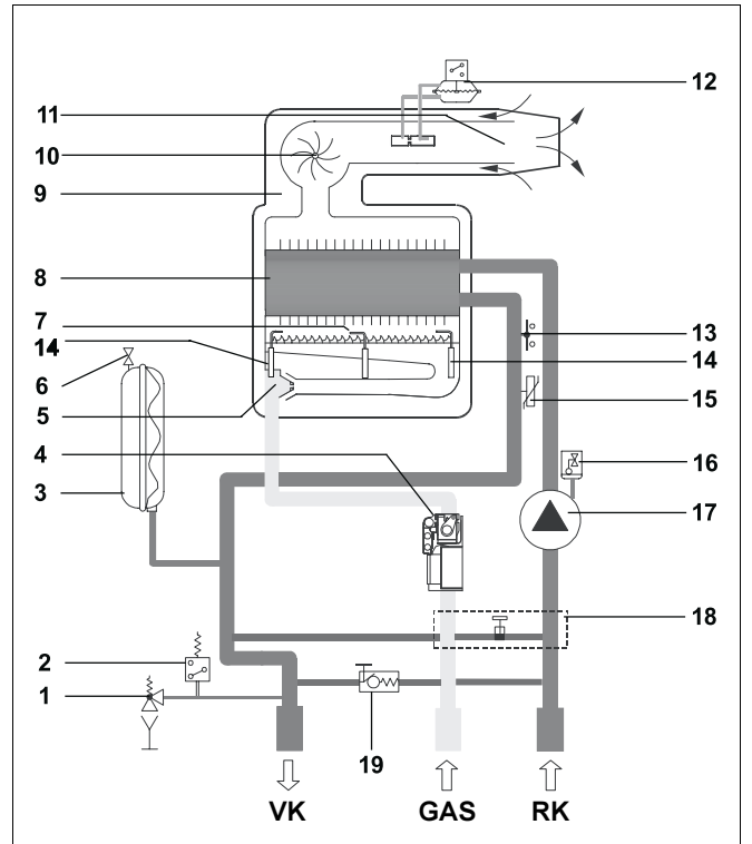
Şekil 6 Logamax U012-24
