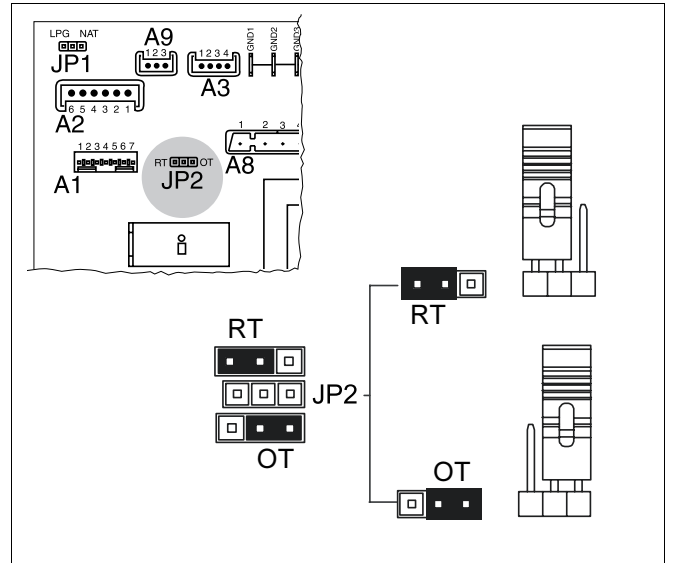
Şekil 42 Oda termostatu tipinin ayarlanması
