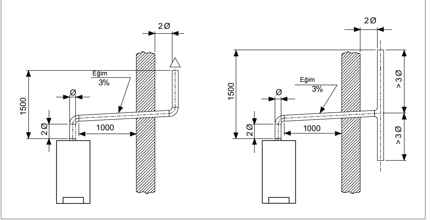
Şekil 10 Baca sistemleri (ölçüler mm)
