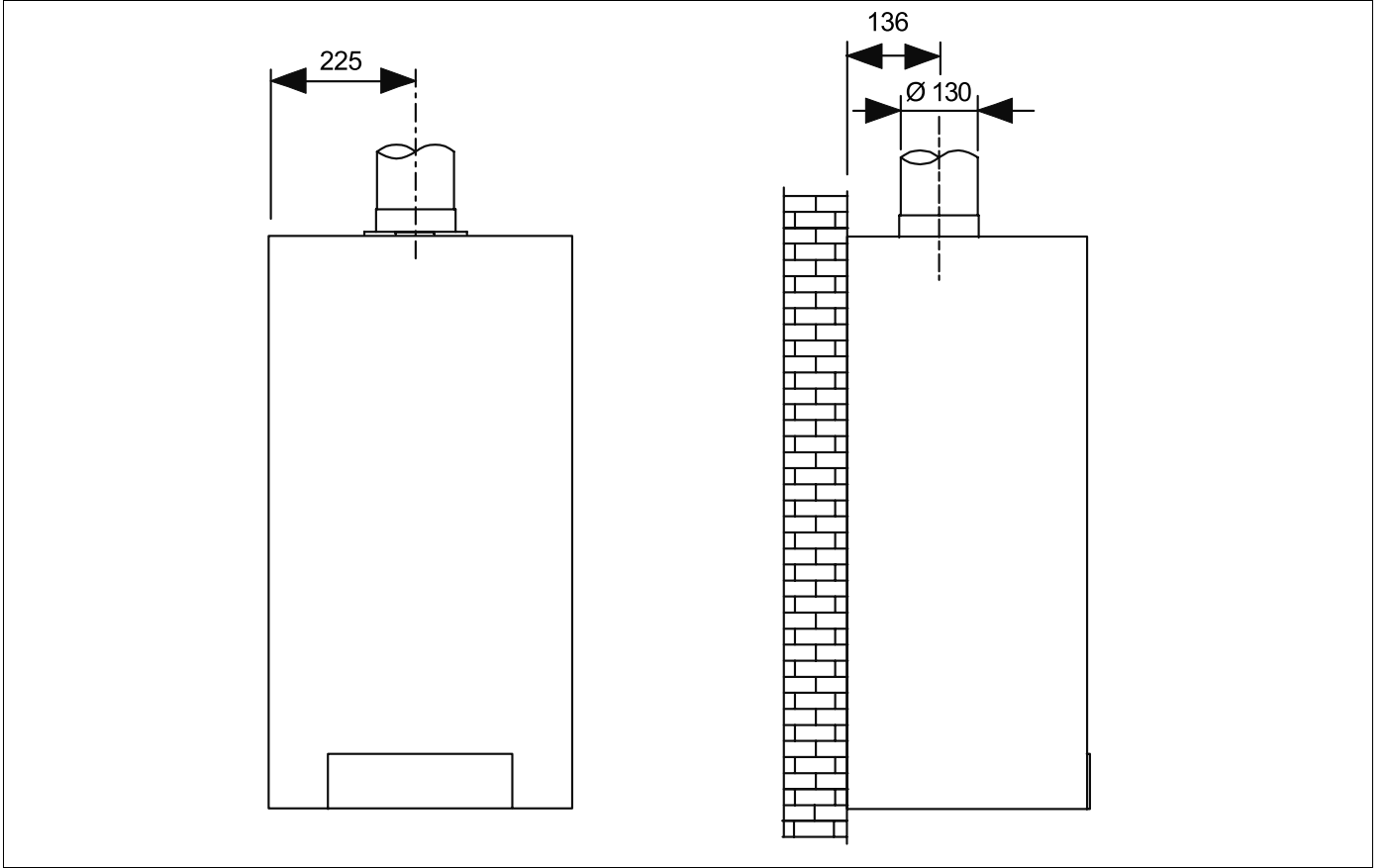
Şekil 11 Baca gazı hattının bağlantı ölçüleri (ölçüler mm)
