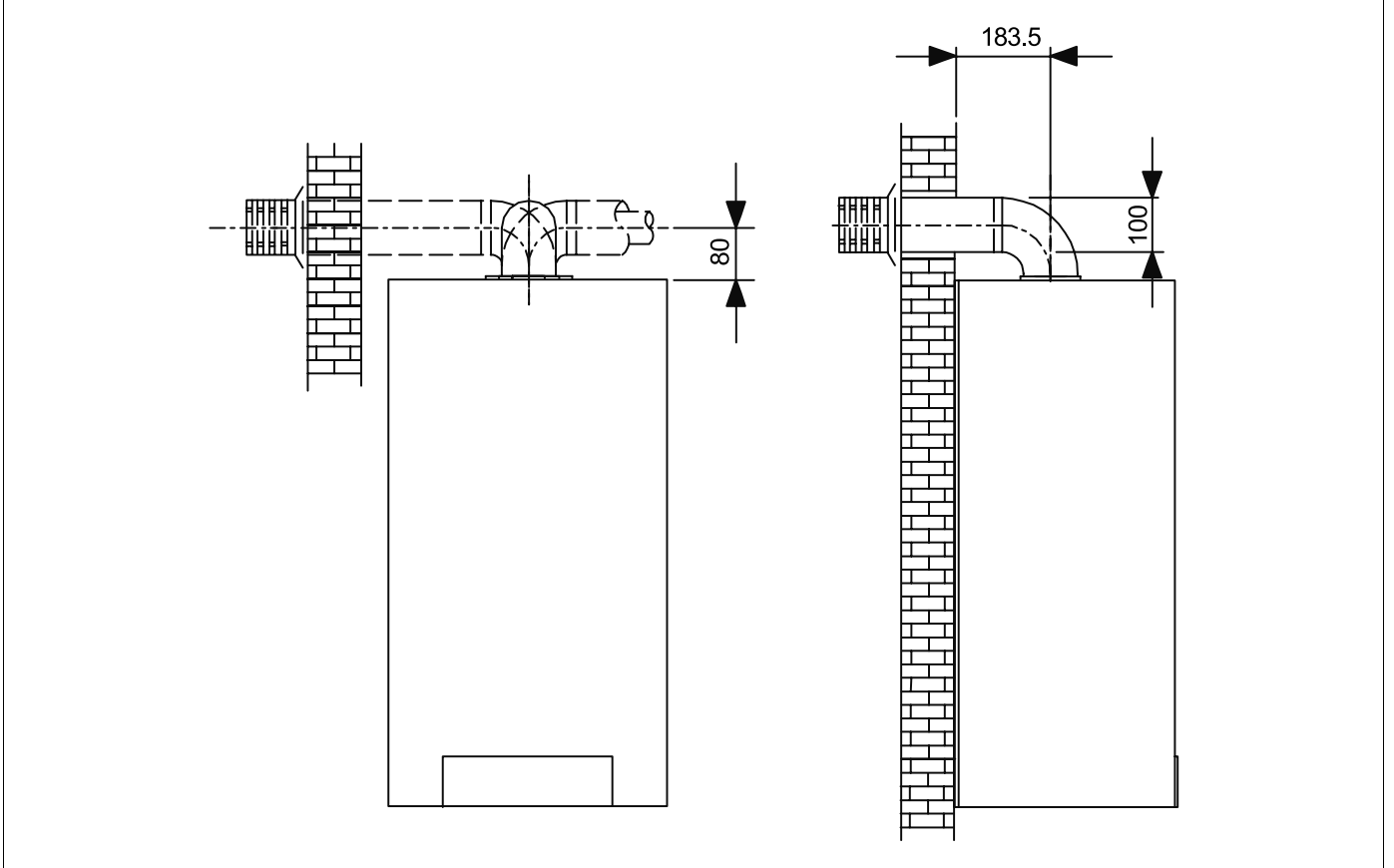
Şekil 21 Eş eksenli baca gazı hattının bağlantı ölçüleri (ölçüler mm)
