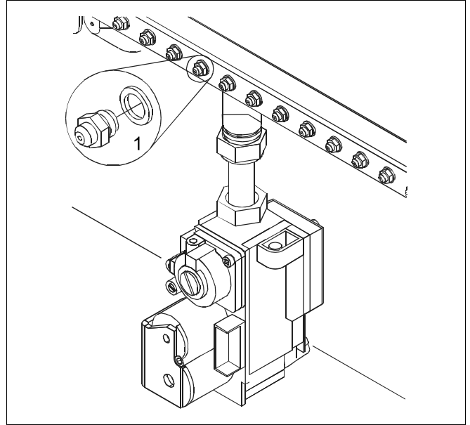
Şekil 48 Memelerin değiştirilmesi
