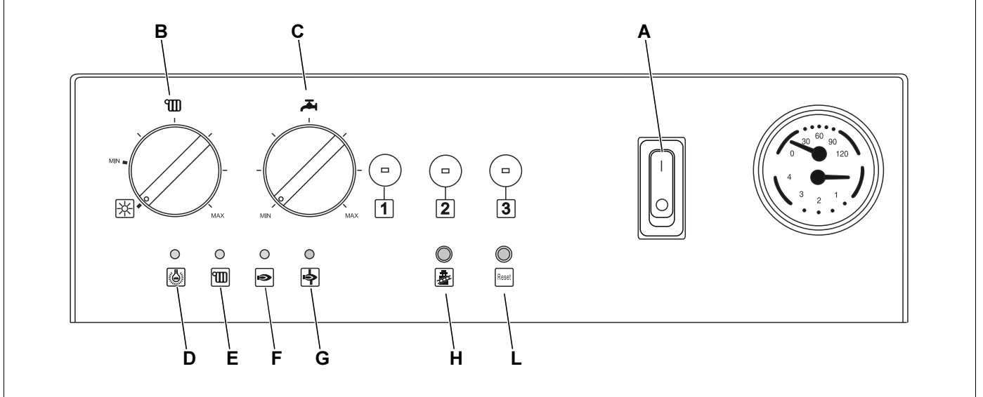
Şekil 55 Kullanma ünitesi
