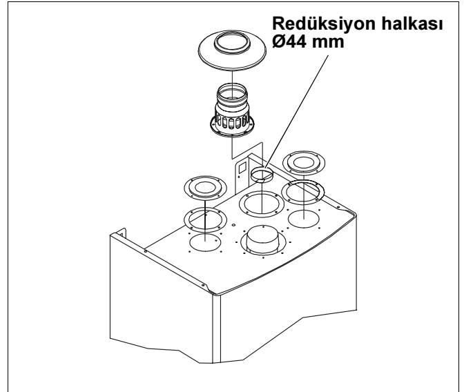
Şekil 14 Redüksiyon halkasının ve adaptörünün montajı
