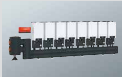
Vitodens 200-W - 8'li kaskad sistem (1200 kW)
