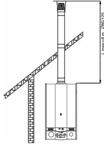
Dikey Hermetik Baca Uygulaması (Dirsekiz Lmax, Mesafesi : 8m, Ø80/125)
