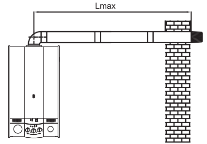
Yatay Hermetik Baca Uygulaması (Tek Dirsekiz Lmax, Mesafesi : 3 m, Ø60/100) (Tek Dirsekiz Lmax, Mesafesi : 6 m, Ø80/125)
